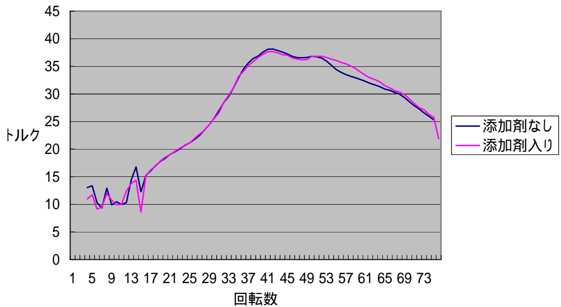
シャーシダイナモによる出力計測
